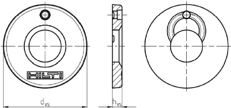
Podkładka Hilti do wypełniania
