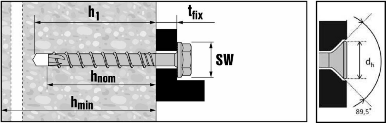
Parametry montażowe dla kotwy HUS3-H oraz -C
