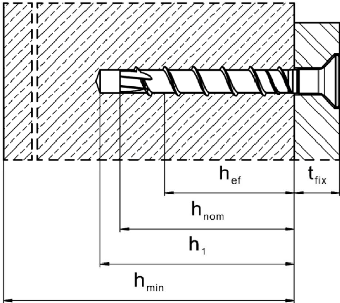
HUS3-C (kotwa w konfiguracji z łbem stożkowym wpuszczanym, rozmiary 6, 8 oraz 10)
