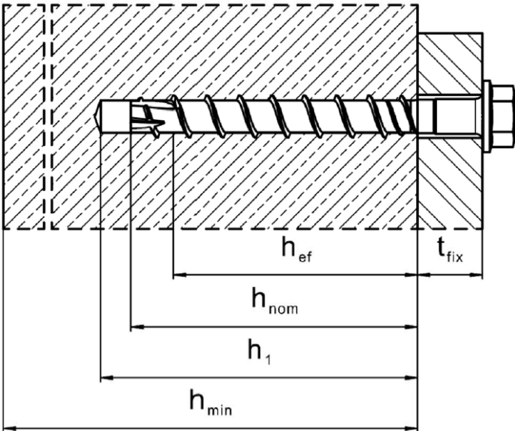
HUS3-H (kotwa w konfiguracji z łbem sześciokątnym, rozmiary 6, 8, 10 oraz 14) HUS3-HF (kotwa w konfiguracji z łbem sześciokątnym, rozmiary 8, 10 oraz 14)
