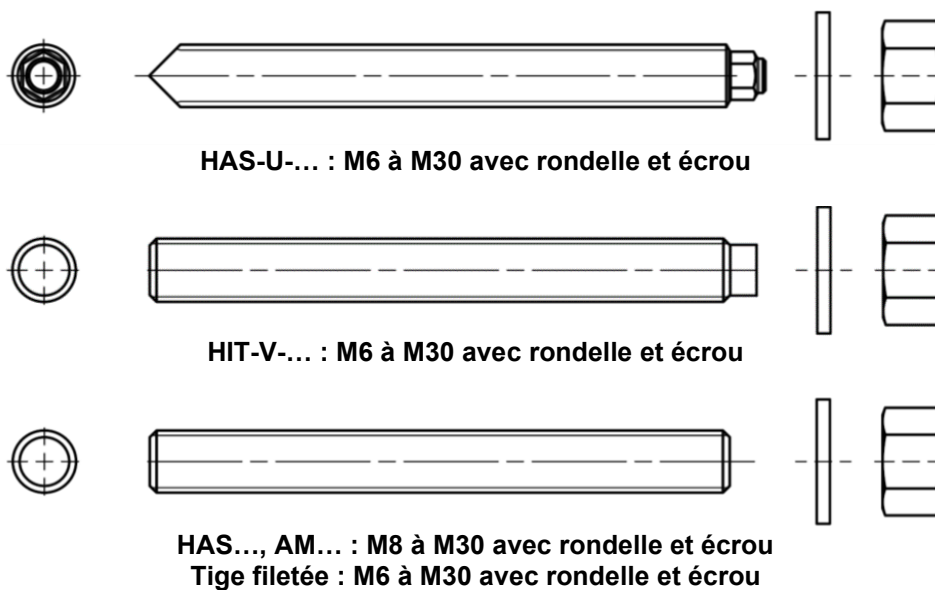
Figure 3 : Élément en acier – tige filetée ; 6 \text{ mm} \leq d \leq 30 \text{ mm}
